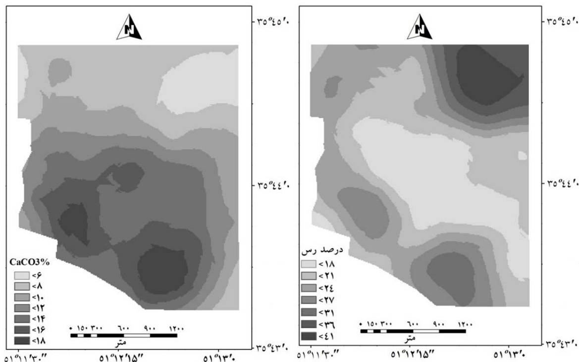
شکل ۲. نقشه‌های تغییرات مکانی مقادیر کرنات کلسیم معادل و رس با استفاده از روش کریجینگ
